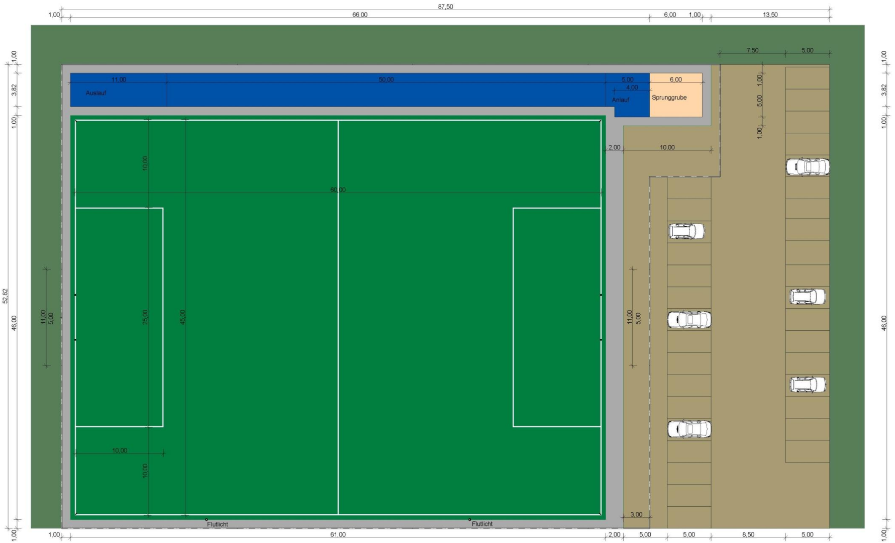
Umgestaltung des Sportplatzes Schwalmtal-Brauerschwend M.: 1/200
